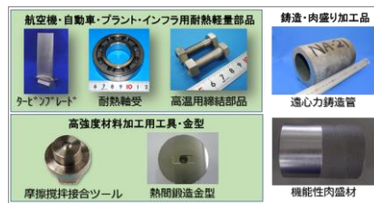
航空機・自動車・プラント・インフラ用耐熱軽量部品 9-ピツアレド 耐熱軸受 高温用締結部品 遠心力鋳造管 高強度材料加工用工具・金型 摩擦攪拌接合ツール 熱間鍛造金型 機能性肉盛材 高温に強いNi基超々合金 (大阪府立大学)
